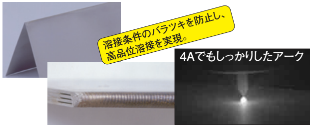
4Aでもしっかりしたアーク (電極:2.4mm 角度:30° 母材-電極間:0.5mm)
